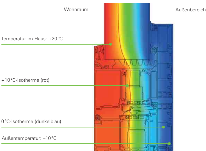
Querschnitt einer hochwärmege­däm­mten Aluminium Haustür von Schüco. Der Isothermenverlauf zeigt: Trotz der Minusgrade außen herrscht auch direkt an der Haustür eine angenehme Innentempe­ratur
