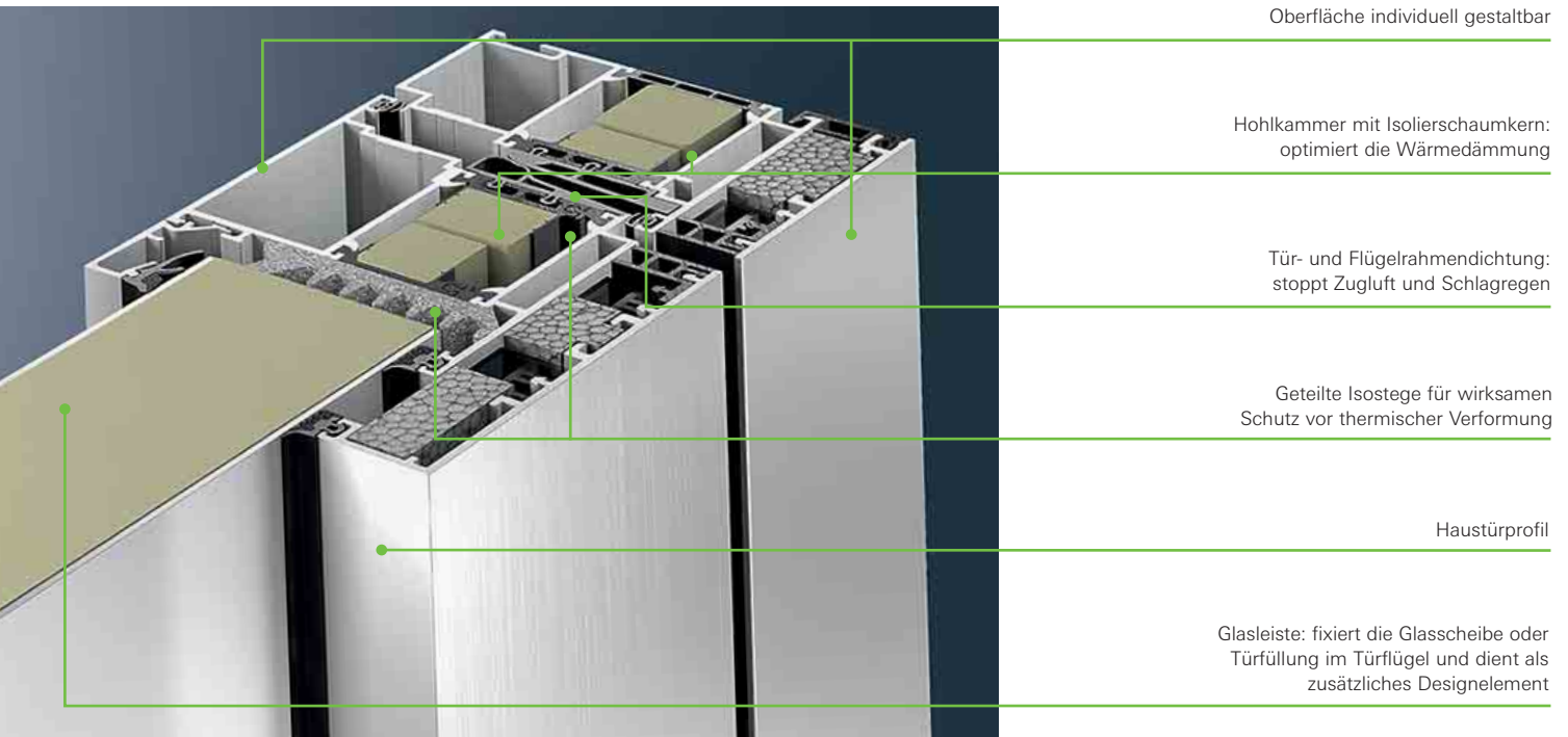
Passivhaus-zertifizierte Wärmedämmung: Schüco ADS 112 IC (Insulation Cover) mit einem U_T -Wert von 1,0 \text{ W}/(\text{m}^2\text{K}) = Dämmwert des Türrahmens
